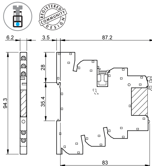
Tipo 39.30/39.30.3 39.31/39.31.3 Borne de jaula
