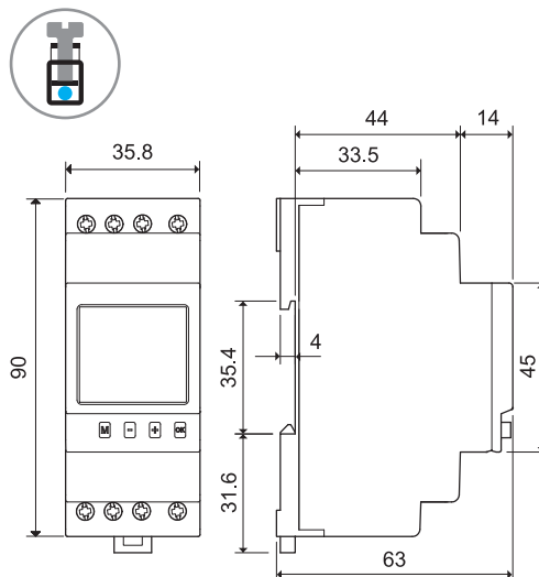
12.51/12.81 Borne de jaula
