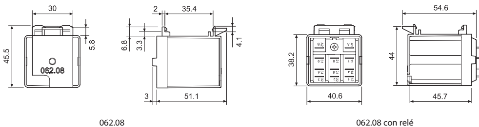
062.08 con relé
