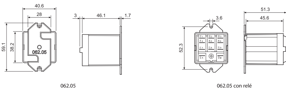
062.05 con relé
