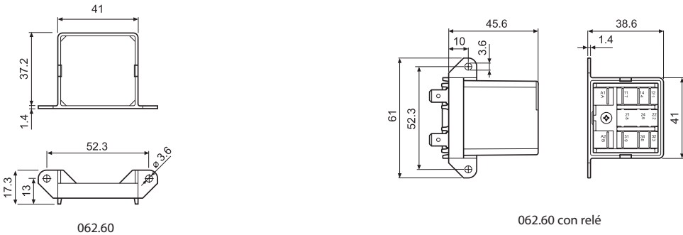
062.60 con relé
