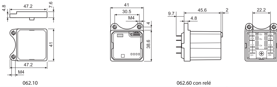
062.60 con relé
