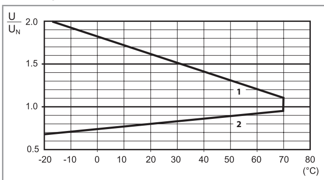
R 56 - Campo de funcionamiento de la bobina DC en función de la temperatura ambiente - 4 contactos conmutados
