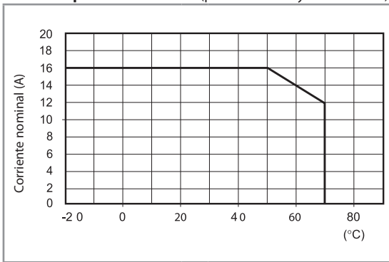
L 97 - Corriente de conmutación en función de la temperatura ambiente (para relé 46.61 y zócalo 97.01)
